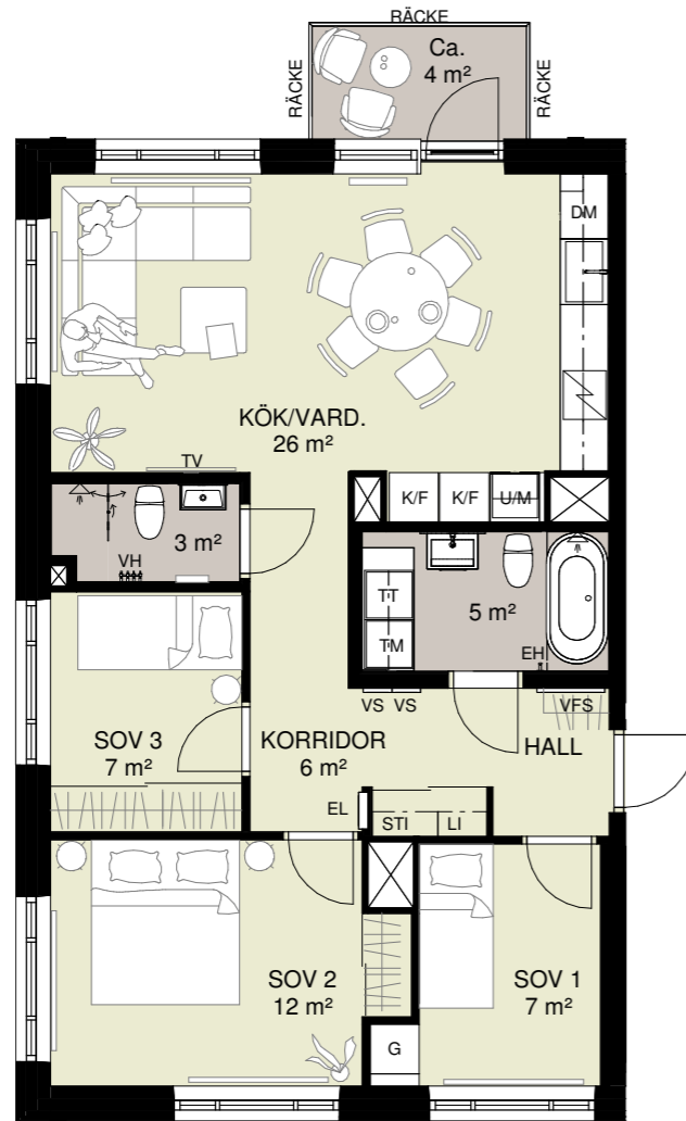
SKALA 1:100
