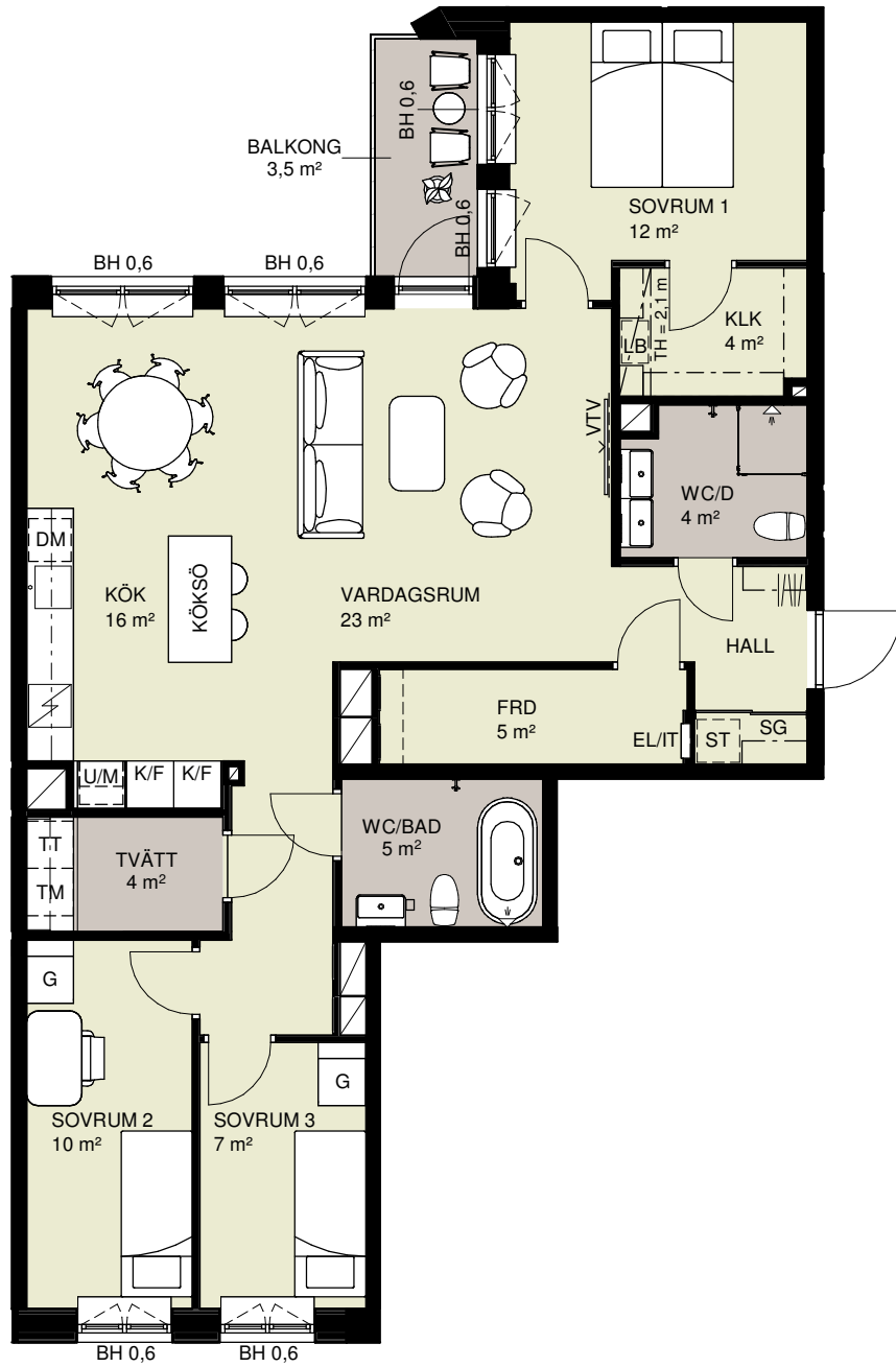
SKALA 1:100
